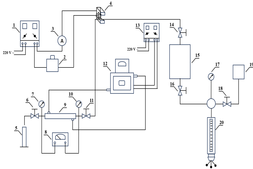
Şəkil 1. Təcrübə qurğusunun sxematik təsviri
