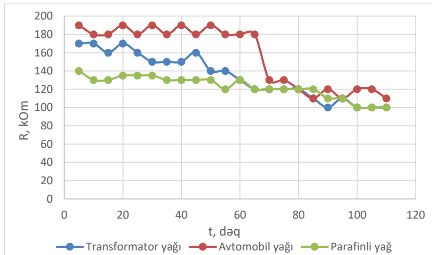
Şəkil 2. Süxurun müqavimətinin zamandan asılılıq qrafiki
