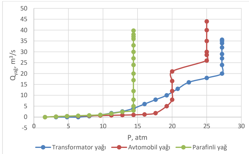
Şəkil 3. Sıxışdırılan yağ miqdarının təzyiqdən asılılıq qrafiki
